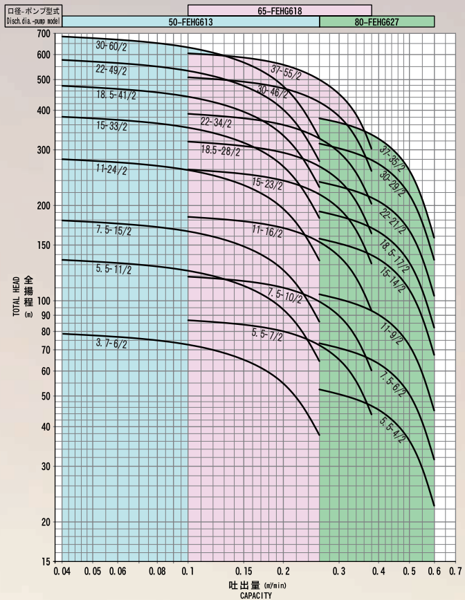
ポンプ選定図FEHG6 50Hz
