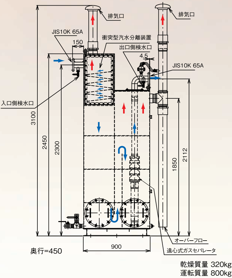
外観寸法図
