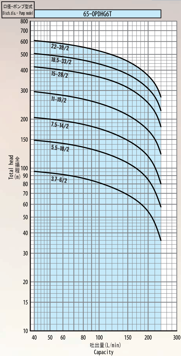
OPDHG6T 60Hz 機種一覧
