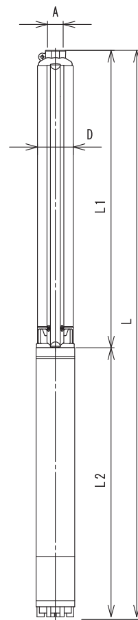
■ 外形図
