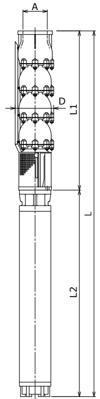
■ 外形図
