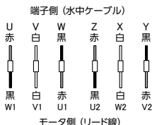
荏原6"モータ + 左回転ポンプ
