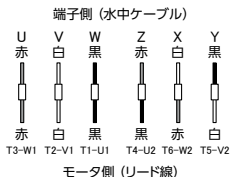
フランクリン6"モータ+右回転ポンプ
