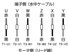
フランクリン6"モータ+左回転ポンプ
