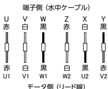
荏原6"モータ + 右回転ポンプ
